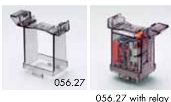
Top 35 mm rail (EN 50022) adaptor for 55.32, 55.33, 55.34
