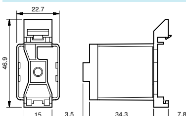
Top 35 mm rail (EN 50022) adaptor for 55.32, 55.33, 55.34
